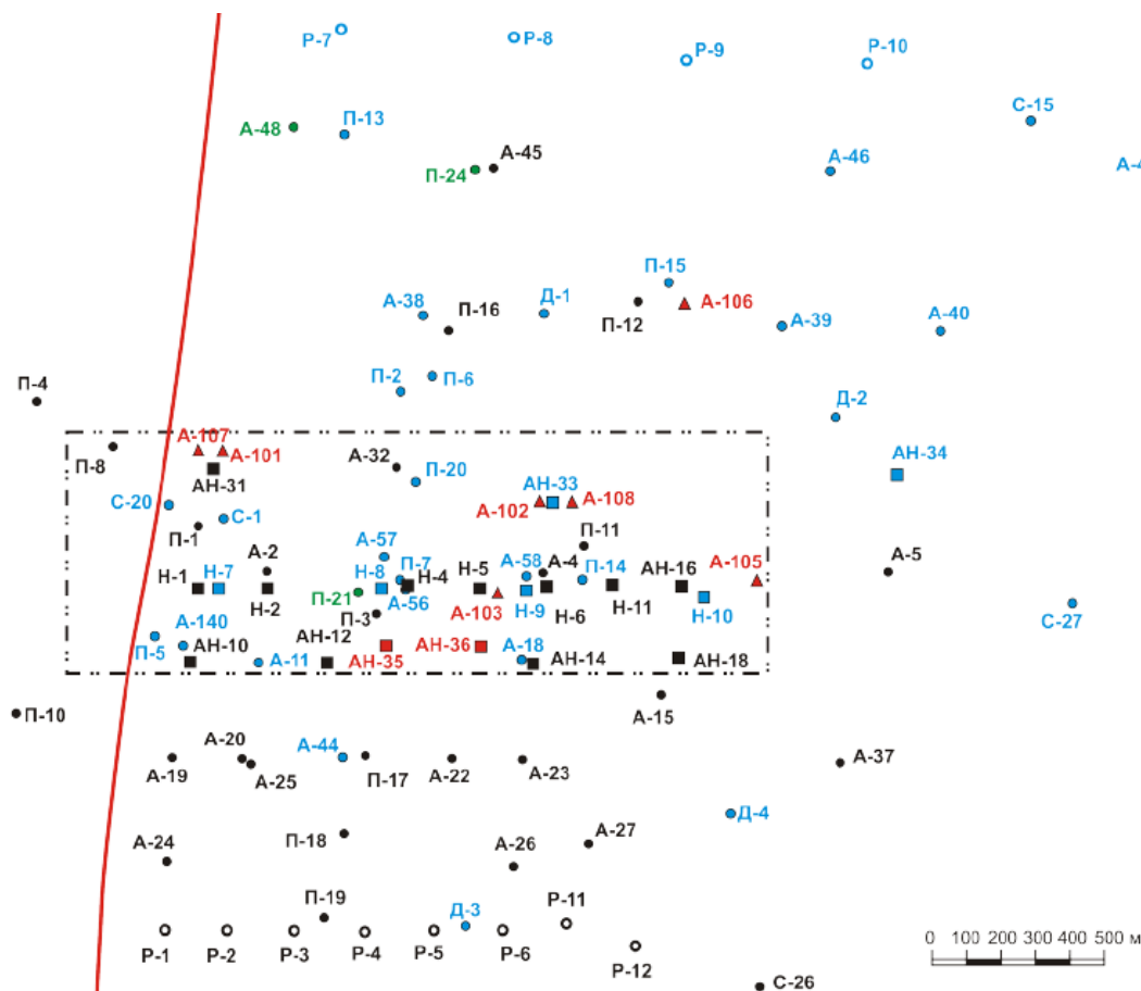
Рисунок 2.3.2 - Схема расположения скважин ПГЗ ЖРО «Полигон «Северный»
