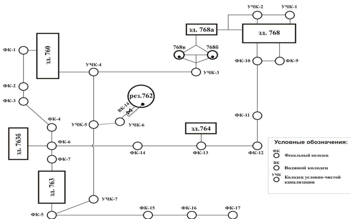
Рисунок 4.4.1 - Схема водоотведения ПГЗ ЖРО
