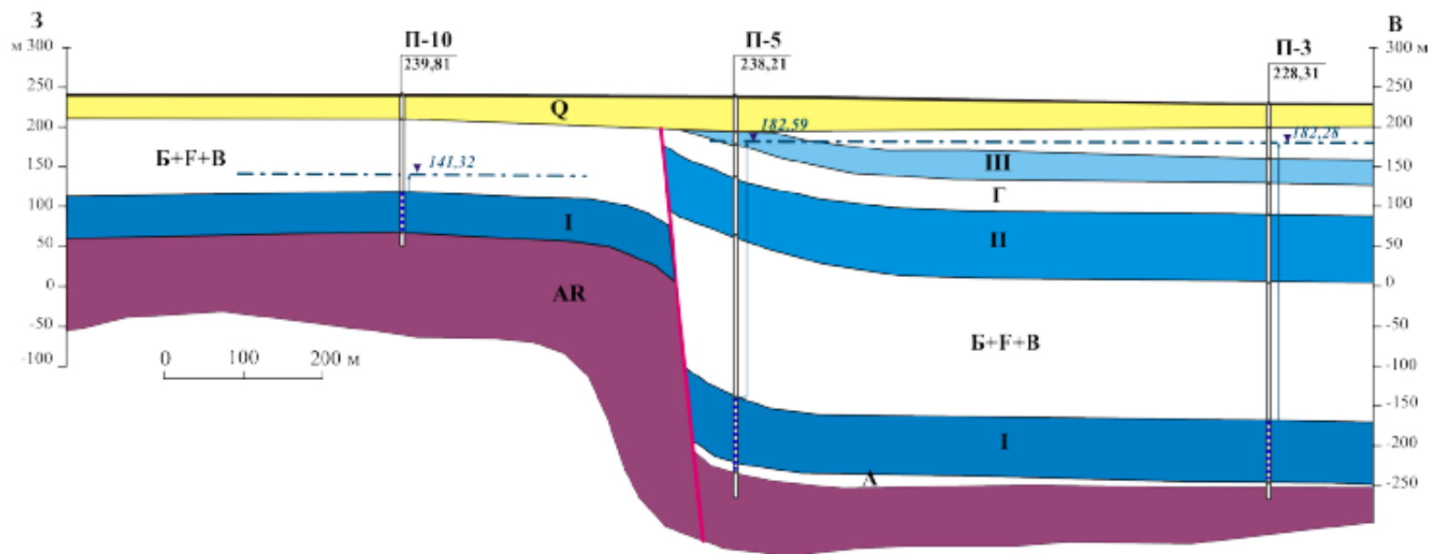
Рисунок 3.1.7 - Схематические геолого-гидрогеологические разрезы
